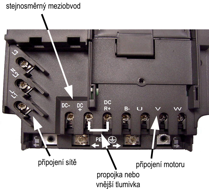
Obr. 7 Silová svorkovnice měničů velikosti C
