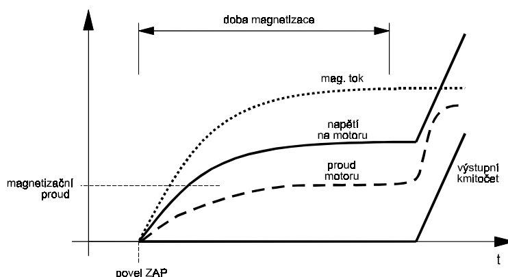
Obr. 62 Pozvolný nárůst magnetizačního napětí
