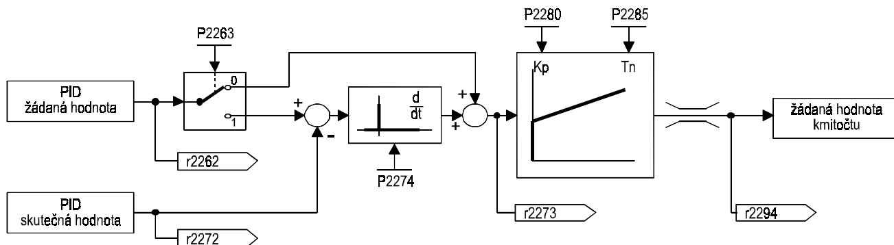
Obr. 84 PID regulátor
