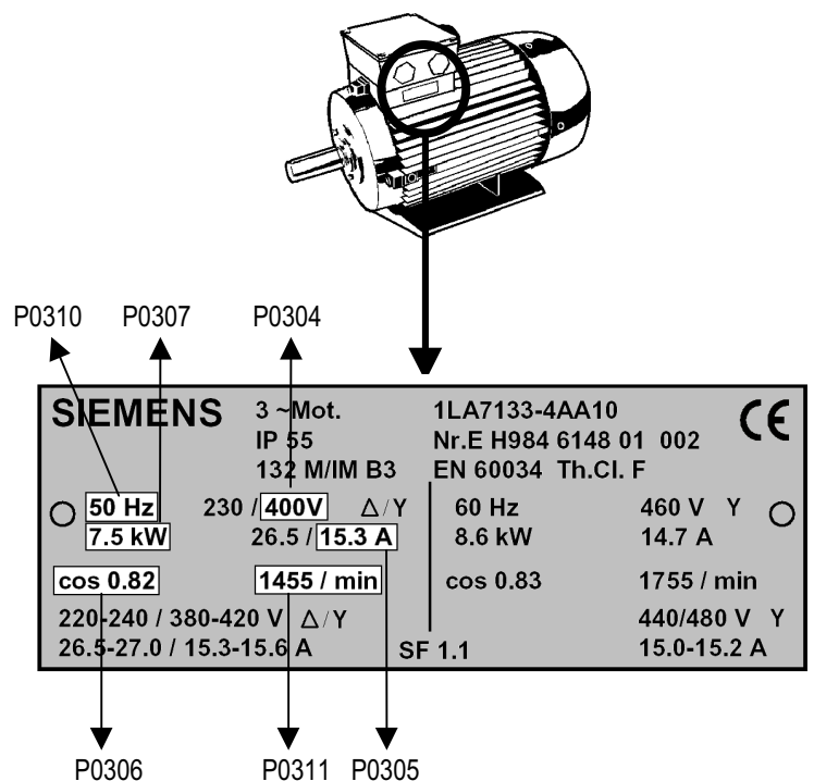
Obr. 25 Výrobní štítek motoru
