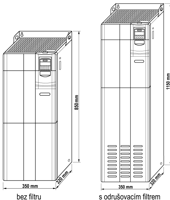
Obr. 3 Náčrtek měničů MICROMASTER 430 a vrtací předpis upevnění měničů
