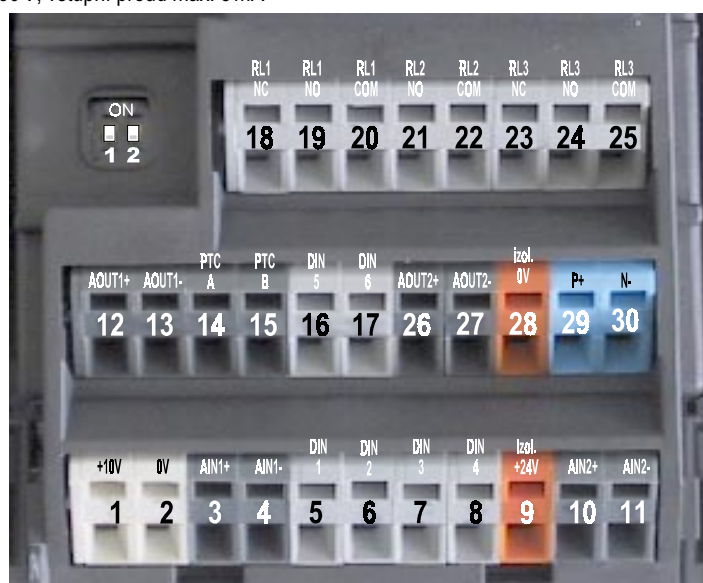
Obr. 14 Řídicí svorkovnice
