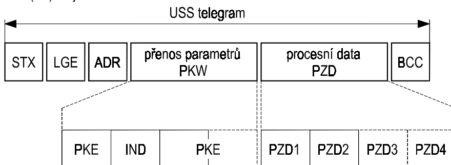
Obr. 63 Komunikační protokol USS
