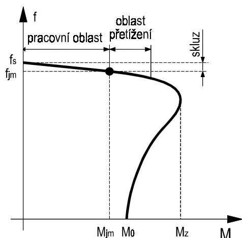
Obr. 58 Momentová charakteristika as. motoru
