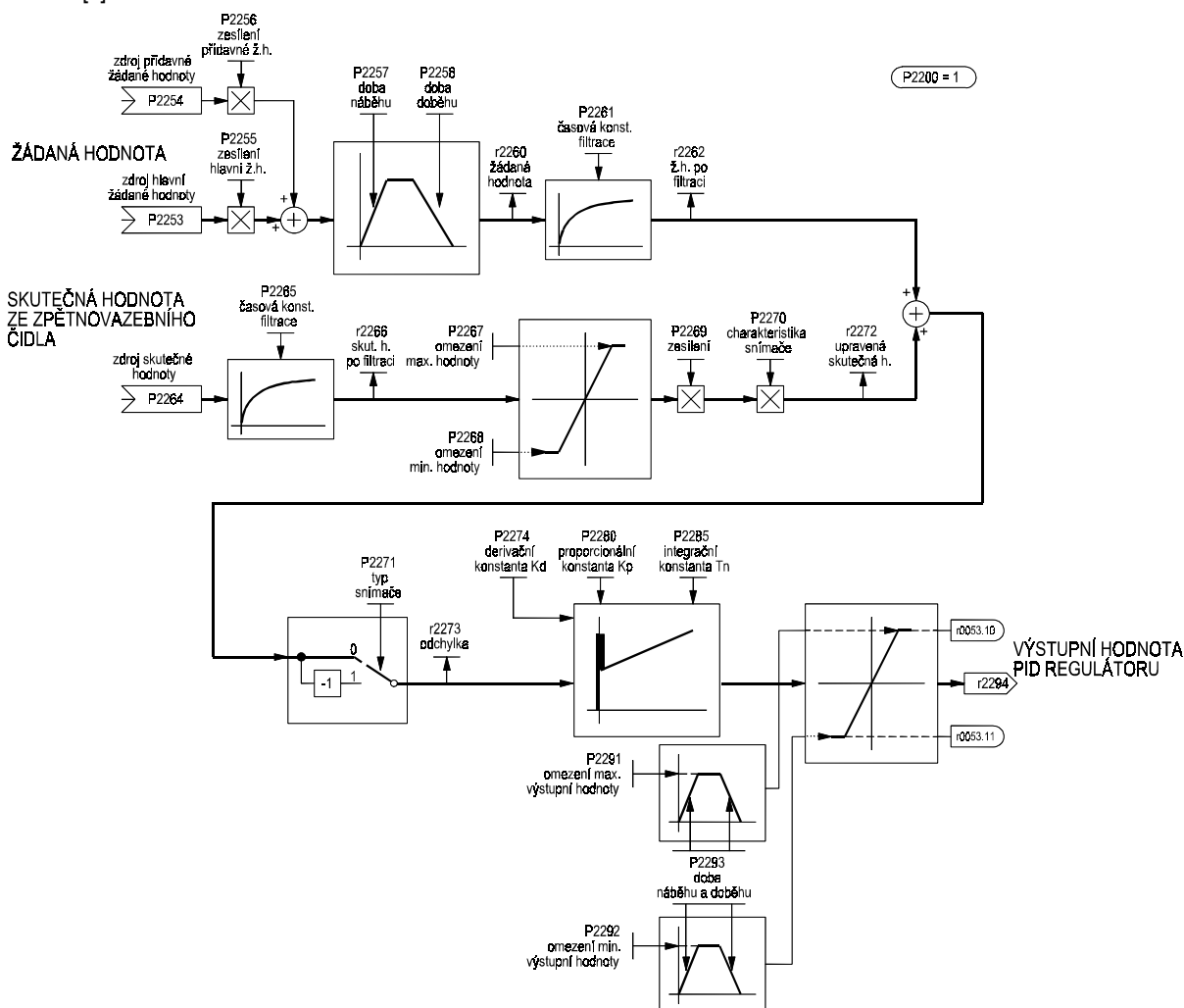
Obr. 81 Schéma technologického PID regulátoru
