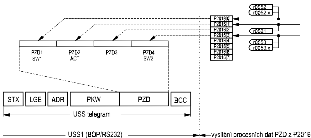
Obr. 67 Vysílání dat PZD přes USS1
