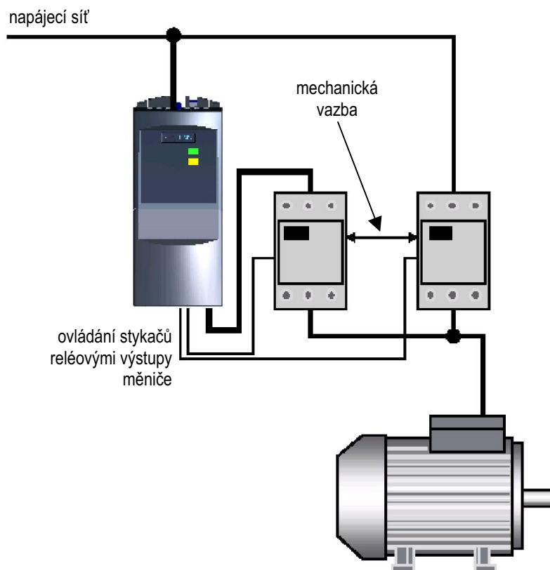
Obr. 26 Principiální schéma napájení motoru z měniče / ze sítě
