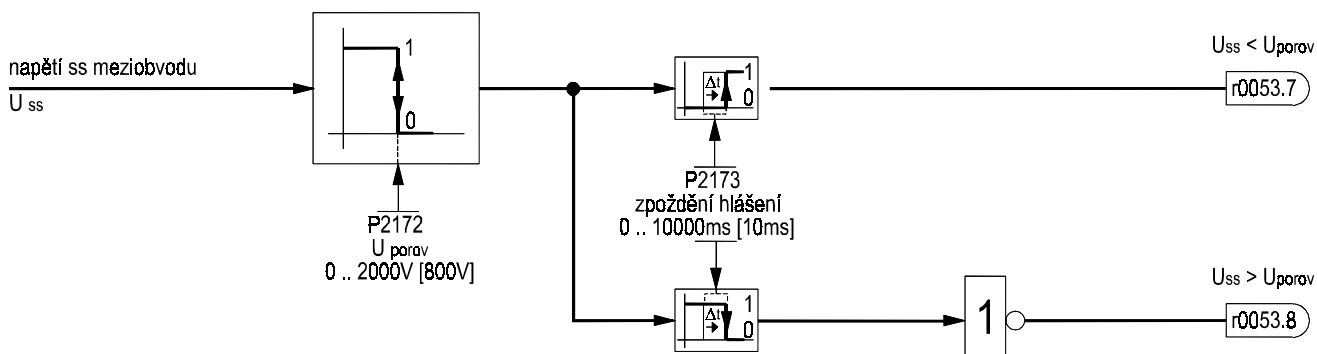
Obr. 78 Porovnání stejnosměrného napětí
