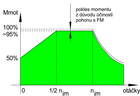
Obr. 17 Redukce zatěžovacího momentu motoru s vlastní ventilací
