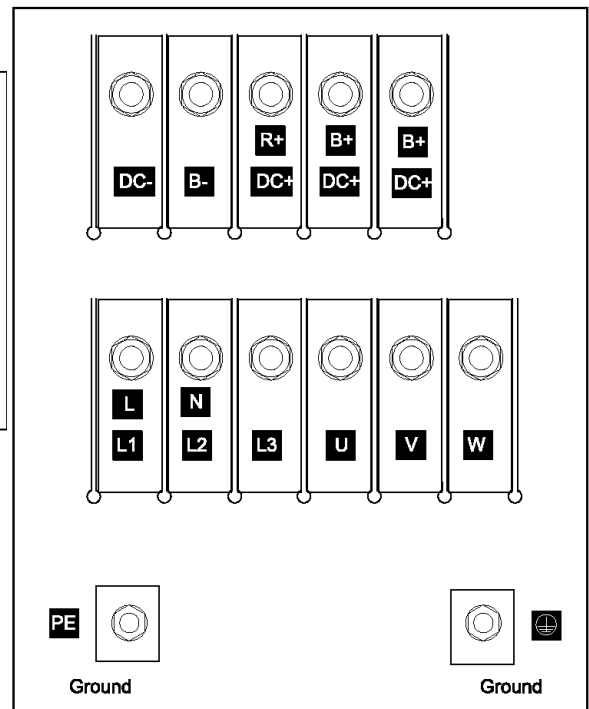
Obr. 7 Silová svorkovnice měničů velikosti C
