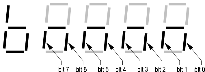
Obr. 32 Zobrazení stavu digitálních vstupů
