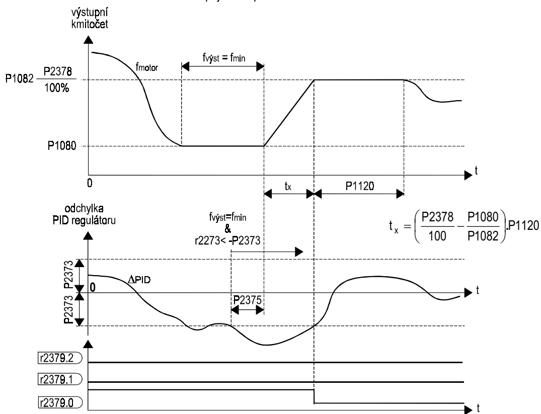
Obr. 86 Odpojení čerpadla v kaskádě
