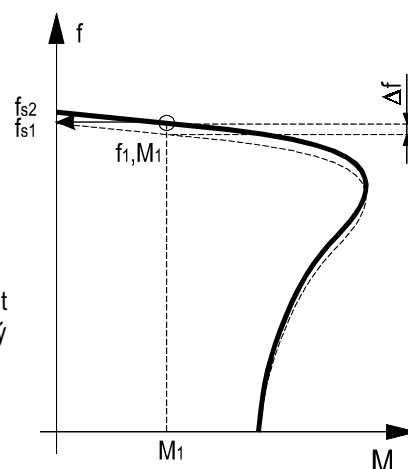
Obr. 59 Kompensace skluzu as. motoru
