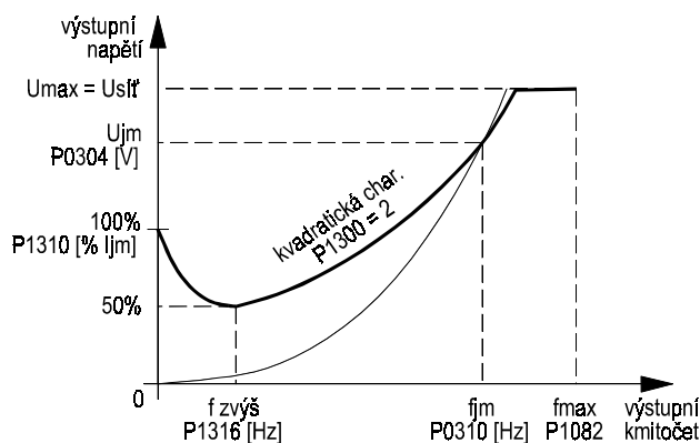
Obr. 55 Kvadratická charakteristika U/f
