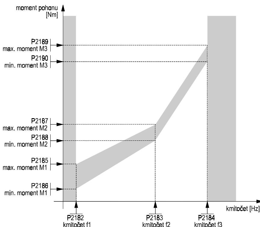
Obr. 80 Režim kontroly momentu
