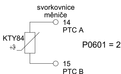
Obr. 19 Zapojení tepl. snímače KTY 84
