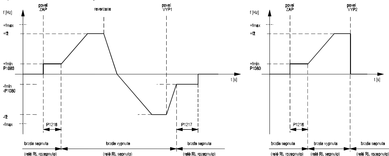
Obr. 51 Způsob ovládání externí brzdy
