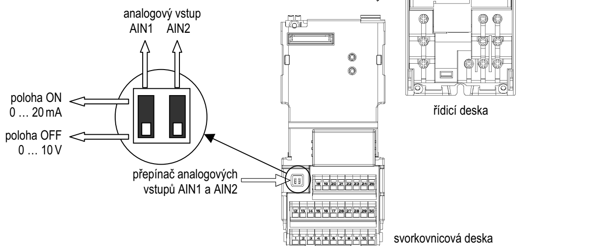
Obr. 16 Význam přepínačů DIP
