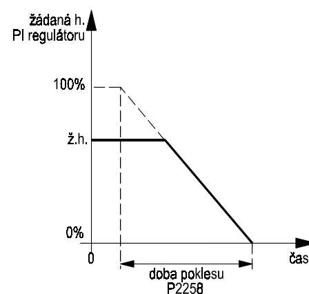
Obr. 83 Doba poklesu žádané hodnoty PID regulátoru
