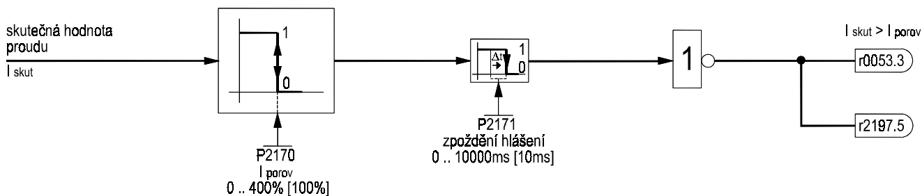
Obr. 77 Porovnání výstupního proudu
