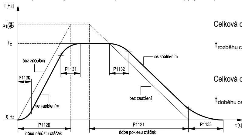
Obr. 46 Zaoblení křivky otáček
