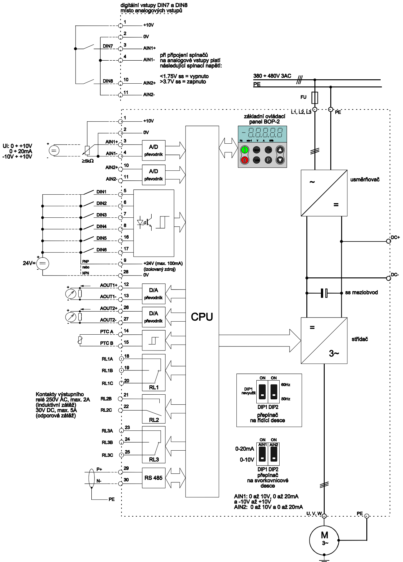
Obr. 20 Blokové schéma měniče
