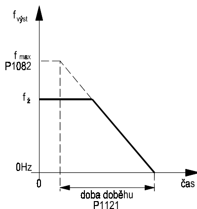
Obr. 45 Doba doběhu motoru
