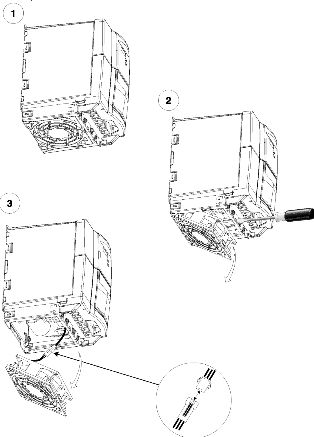
Obr. 88 Demontáž chladičího ventilátoru měniče vel. C
