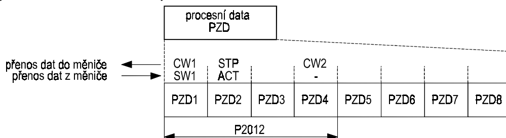
Obr. 64 Přenos procesních dat PZD
