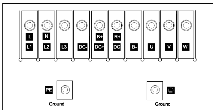
Obr. 8 Silová svorkovnice měničů velikosti D a E
