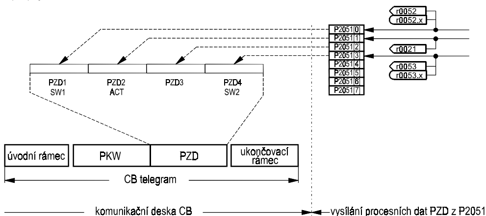
Obr. 71 Vysílání dat PZD přes komunikační desku CB
