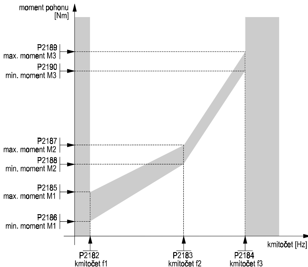
Obr. 27 Režim kontroly momentu
