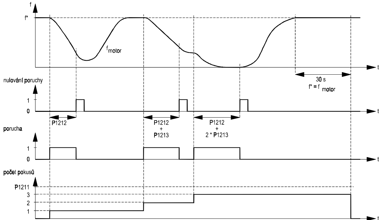
Obr. 50 Automatické opakování restartu pohonu
