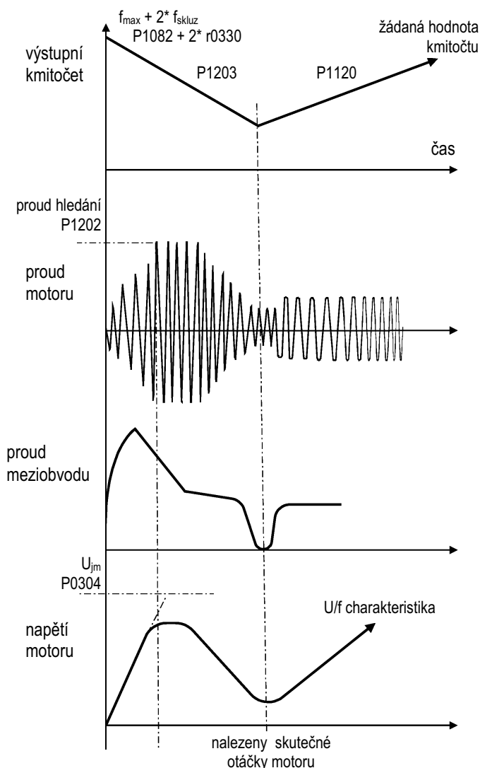
Obr. 48 Synchronizace na otáčející se motor
