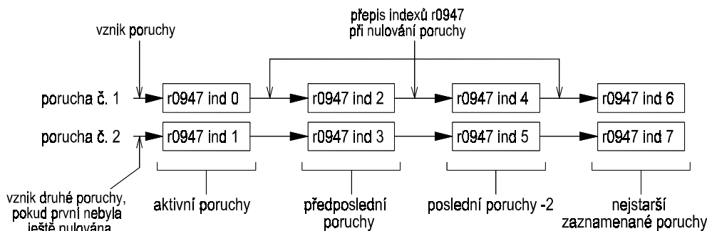
Obr. 41 Paměť poruch
