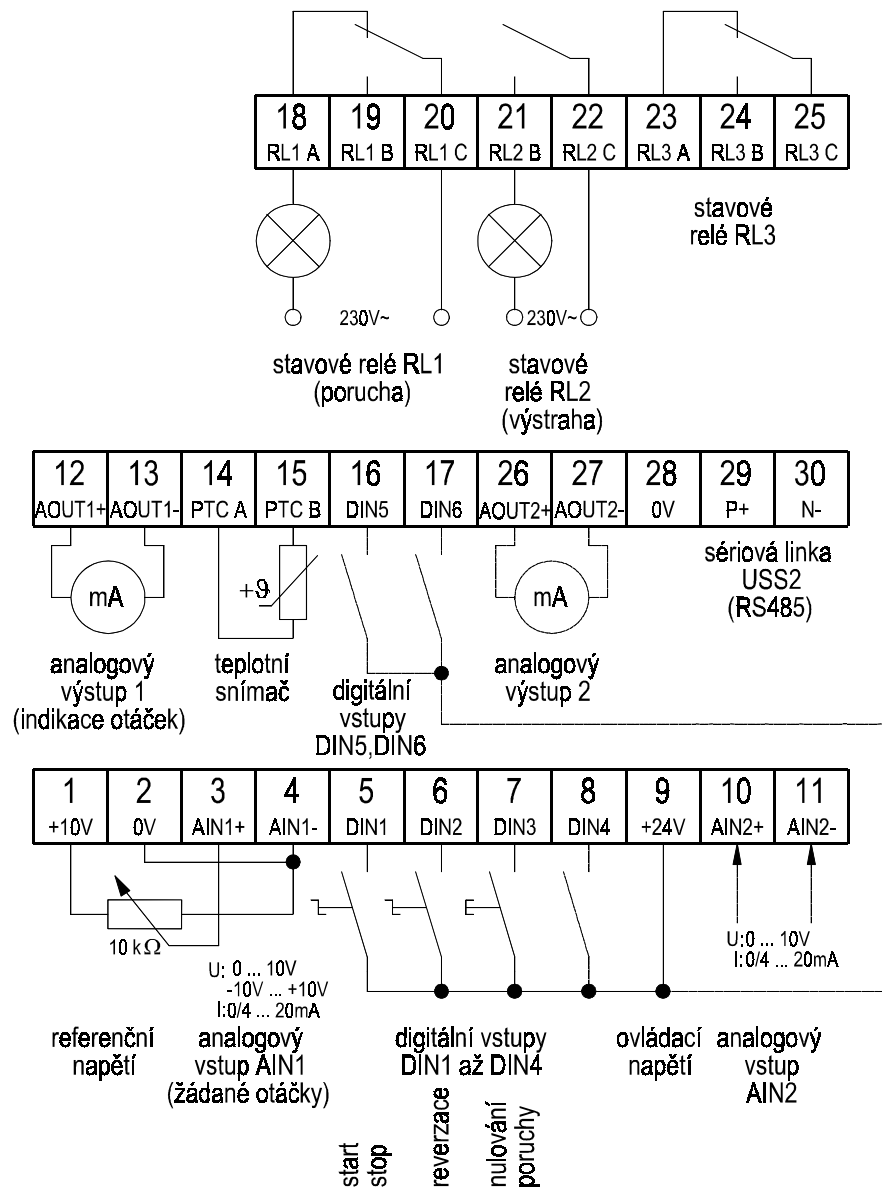
Obr. 24 Význam svorek při továrním nastavení měniče
