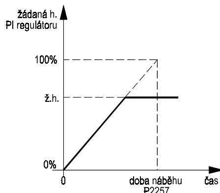
Obr. 82 Doba náběhu žádané hodnoty PID regulátoru
