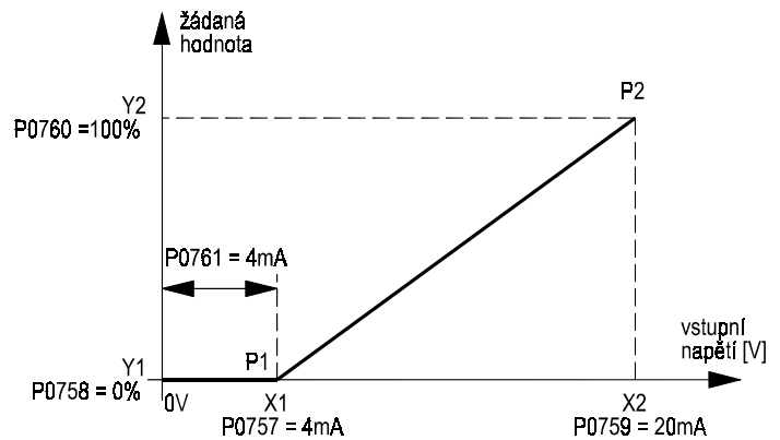
Obr. 35 Nastavení AIN pro proudovou smyčku 4 ÷ 20 mA
