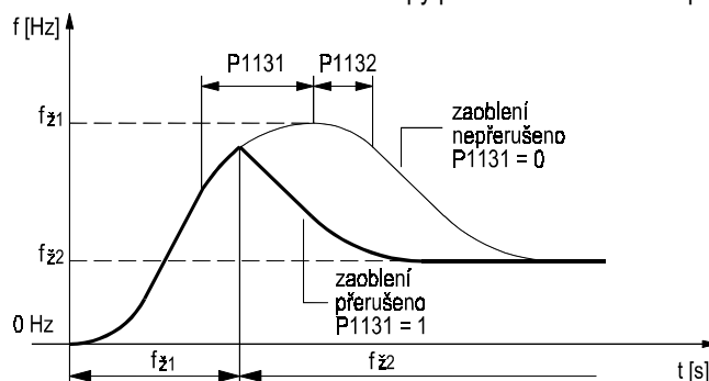
Obr. 47 Způsob zaoblení křivky otáček
