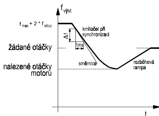
Obr. 49 Rychlost synchronizace na otáčející se motor
