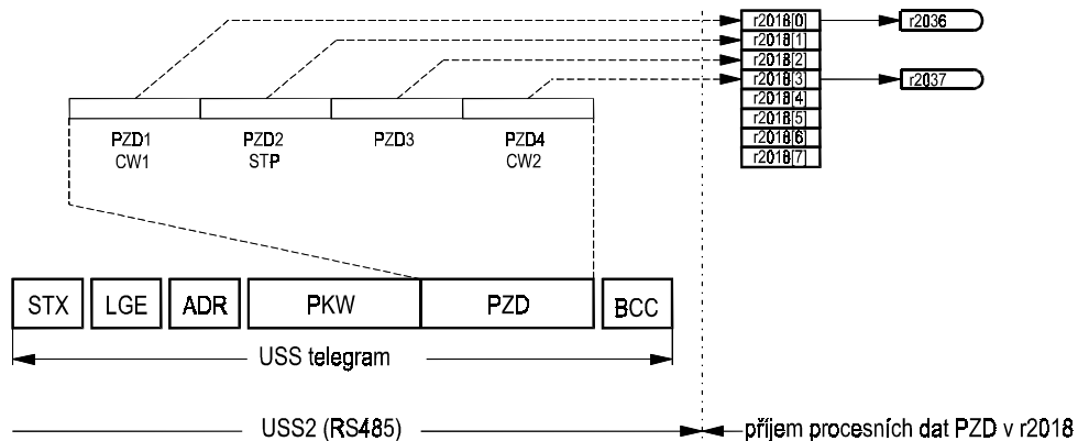
Obr. 68 Příjem dat PZD přes USS2
