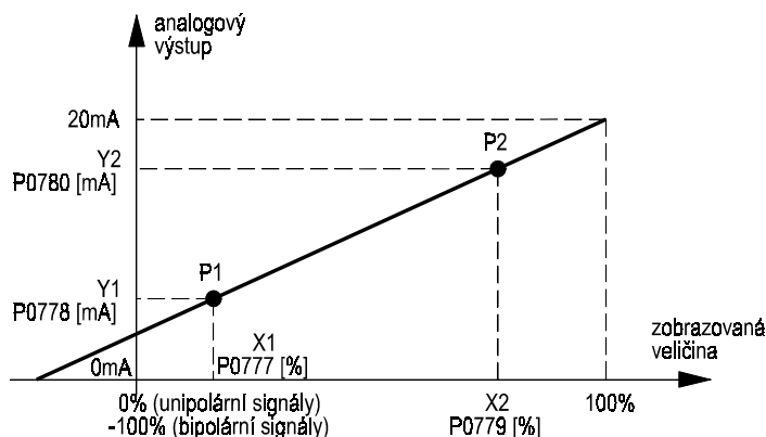
Obr. 37 Normování analogového výstupu AOUT
