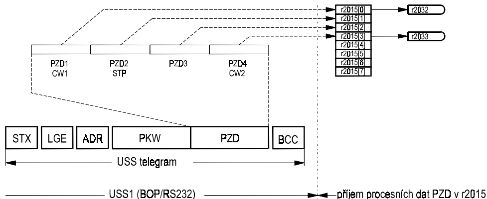
Obr. 66 Příjem dat PZD přes USS1
