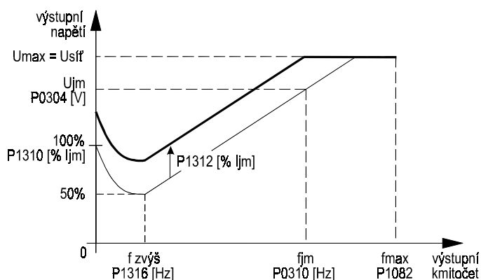
Obr. 56 Posun U/f charakteristiky při rozběhu
