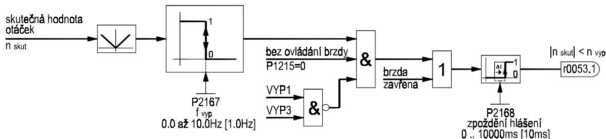
Obr. 76 Kmitočet vypnutí měniče
