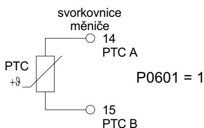
Obr. 18 Zapojení PTC motoru
