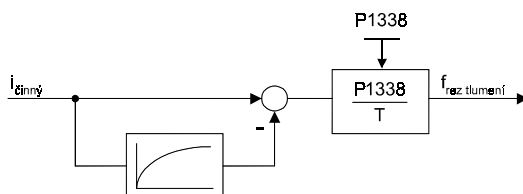
Obr. 60 Rezonanční tlumení
