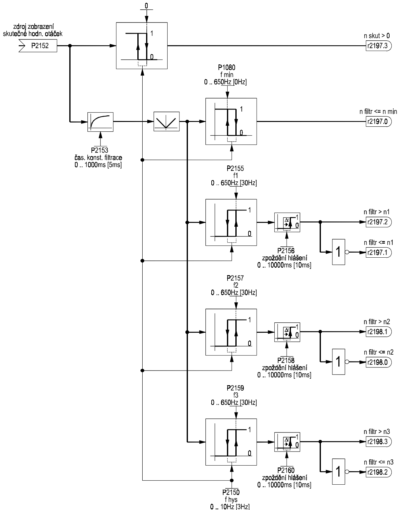
Obr. 73 Porovnání skutečné hodnoty otáček
