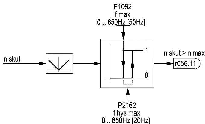
Obr. 74 Porovnání maximální hodnoty otáček
