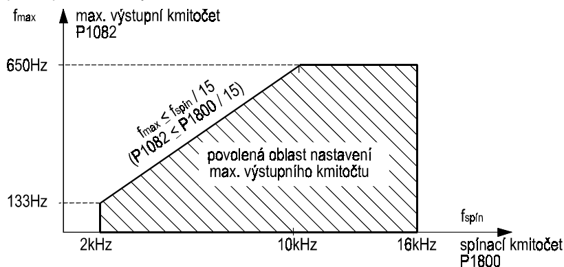
Obr. 42 Max. výstupní kmitočet měniče
