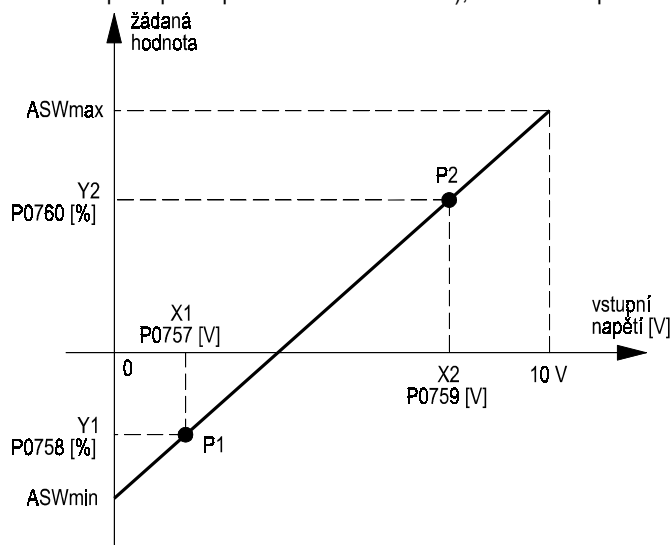
Obr. 34 Normování analogového vstupu AIN
