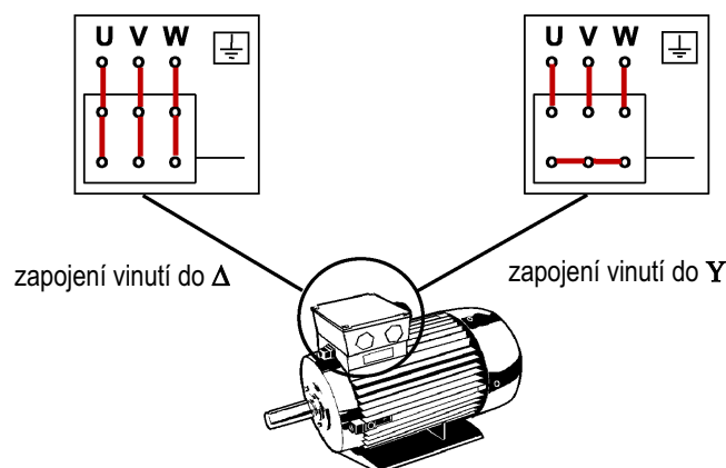
Obr. 10 Zapojení vinutí motoru do trojúhelníku nebo do hvězdy
