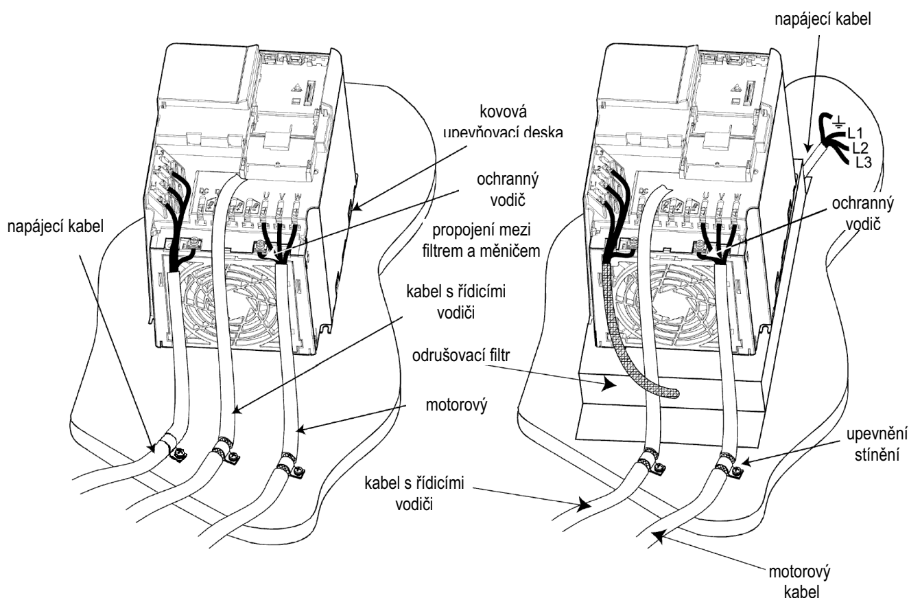
Obr. 21 Způsob propojení měniče z hlediska EMC
