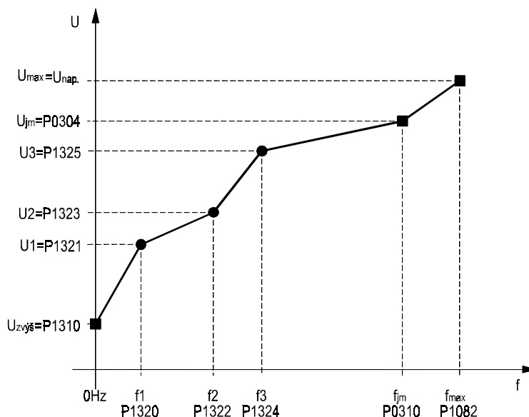
Obr. 57 Vícebodová U/f charakteristika
