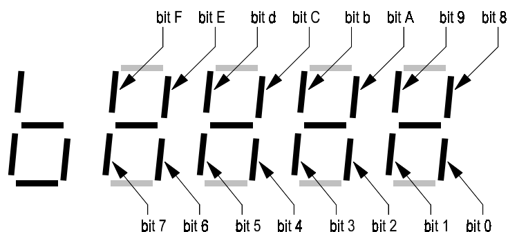
Obr. 30 Zobrazení binárně kódovaných hodnot parametrů
