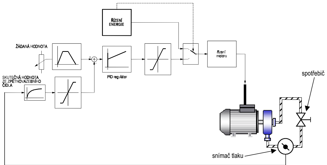
Obr. 29 Principiální schéma režimu úspory energie
