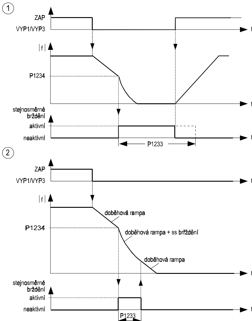
Obr. 52 Stejnoseměrné brždění po povelu VYP1 nebo VYP3
