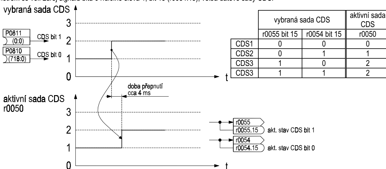
Obr. 38 Přepínání sad CDS
