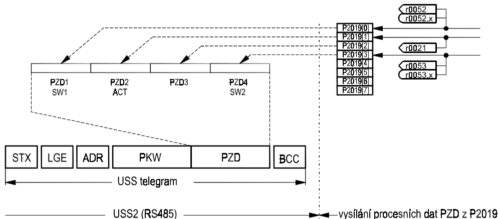
Obr. 69 Vysílání dat PZD přes USS2
