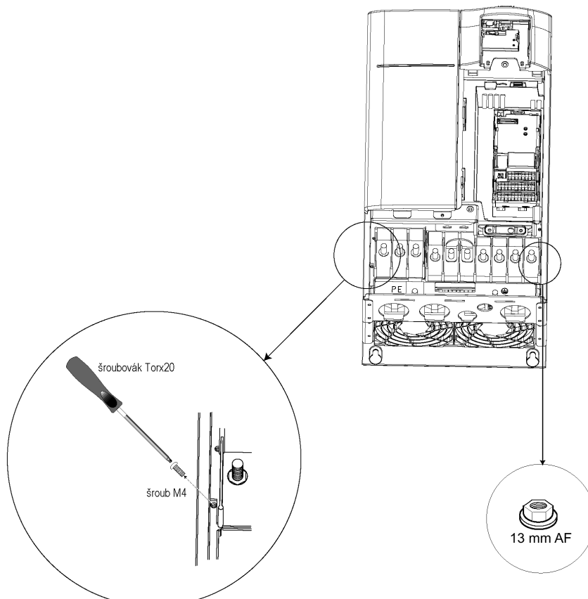
Obr. 5 Odpojení kondenzátoru Y u měničů velikosti D a E
