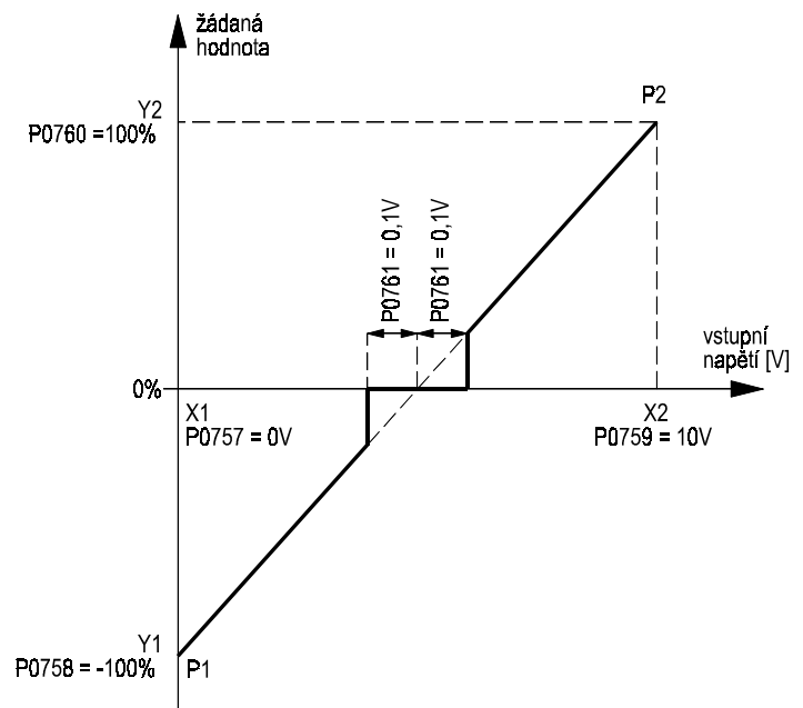
Obr. 36 Nastavení AIN pro zadávání směru otáčení analogovým signálem
