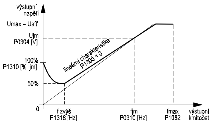
Obr. 54 Lineární charakteristika U/f
