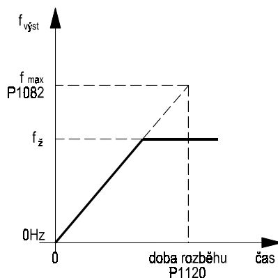
Obr. 44 Doba rozběhu motoru
