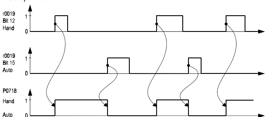
Obr. 31 Přepínání způsobu ovládání HAND / AUTO
