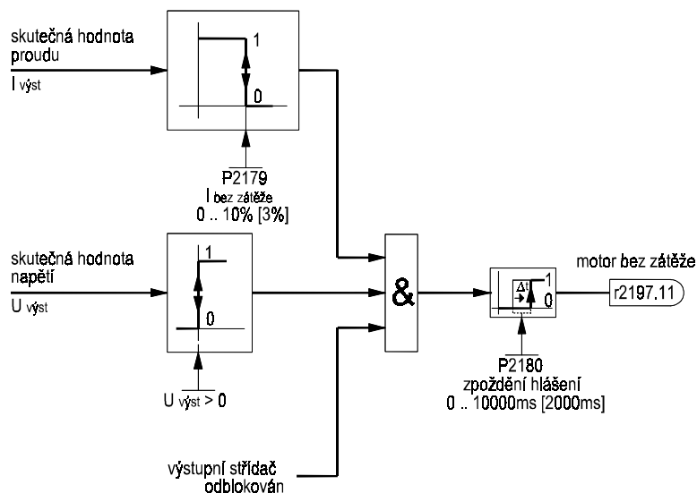
Obr. 79 Hlídkání odlehčení motoru
