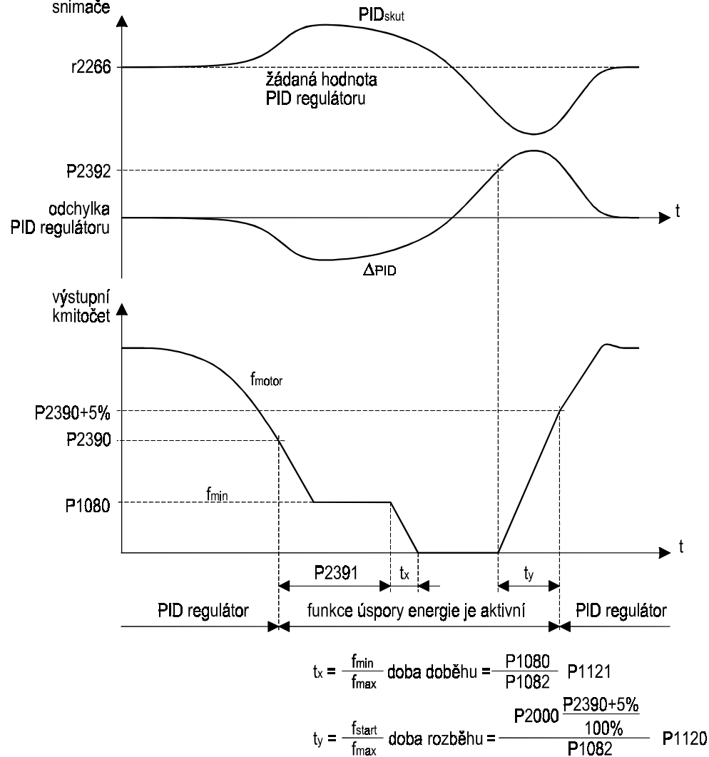
Obr. 87 Režim úspory energie
