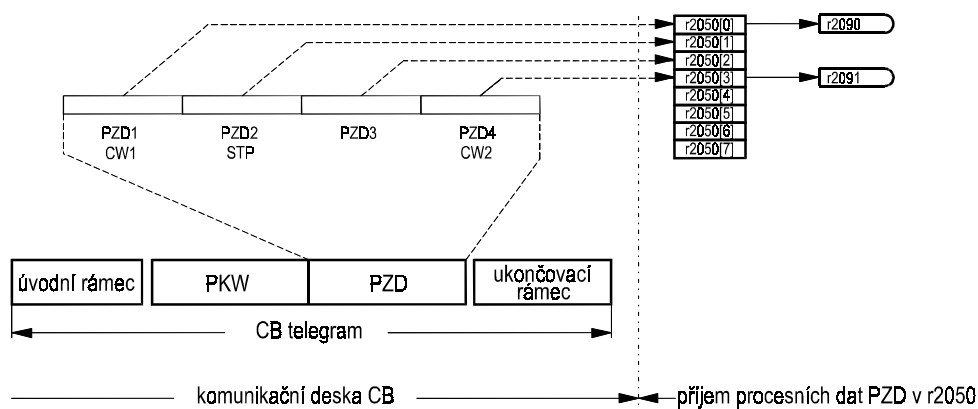
Obr. 70 Přijem dat PZD přes komunikační desku CB
