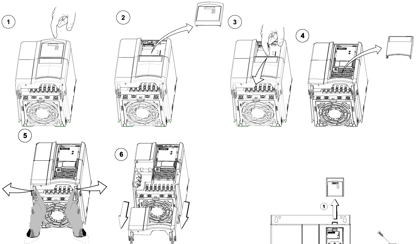
Obr. 11 Odejmutí krytů svorkovnic měniče velikosti C
