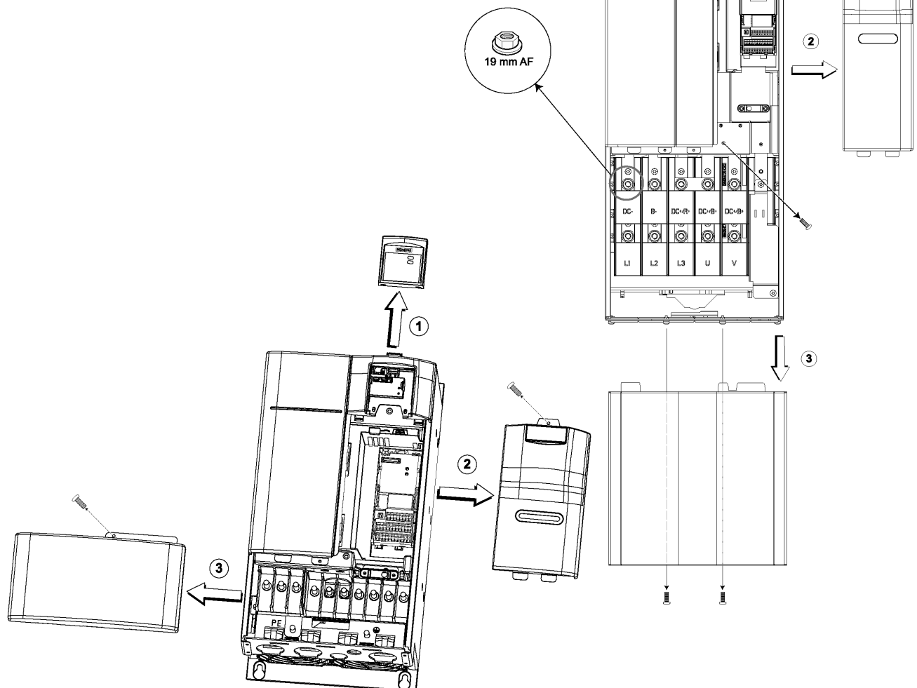
Obr. 12 Odejmutí krytů svorkovnic měniče velikosti D a E
