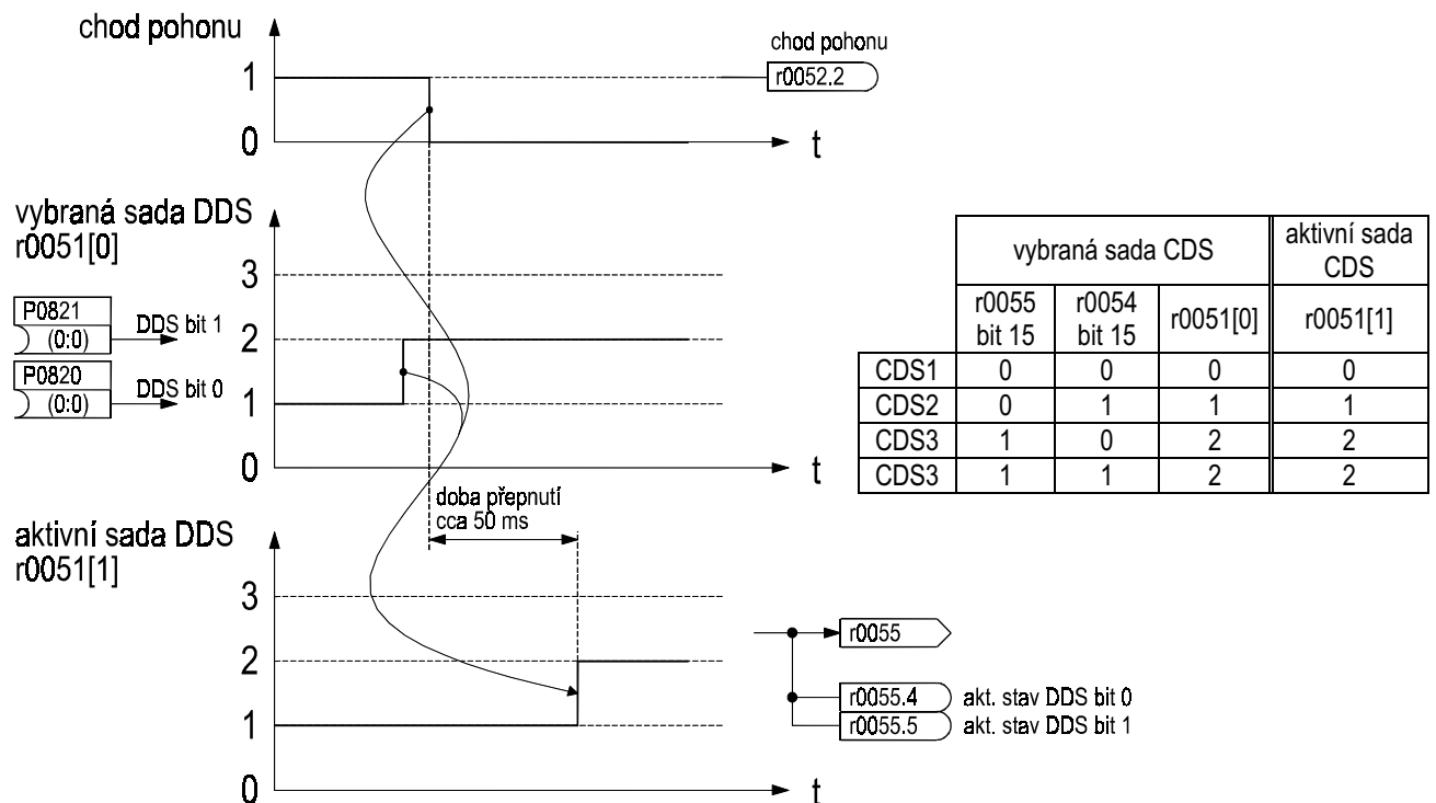
Obr. 39 Přepínání sad DDS
