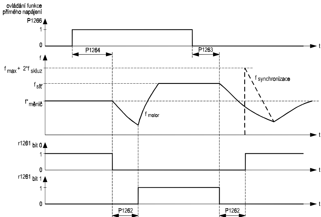
Obr. 53 Funkce přímého napájení motoru
