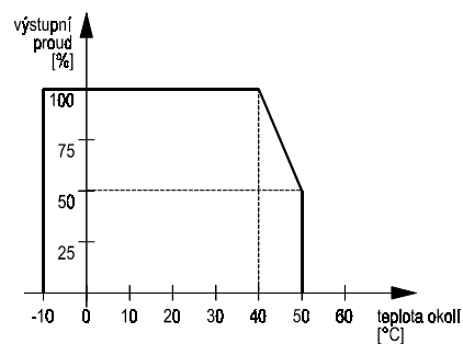
Obr. 1 Graf přípustné provozní teploty měniče
