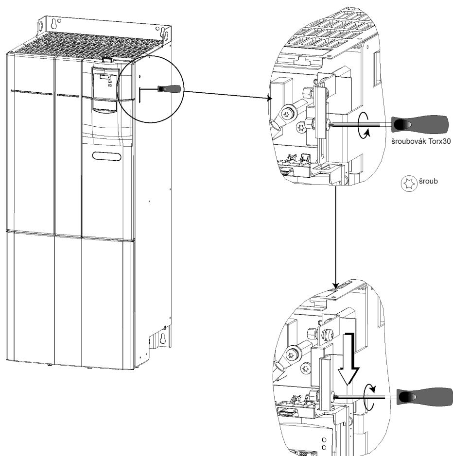
Obr. 6 Odpojení kondenzátoru Y u měniče velikosti F
