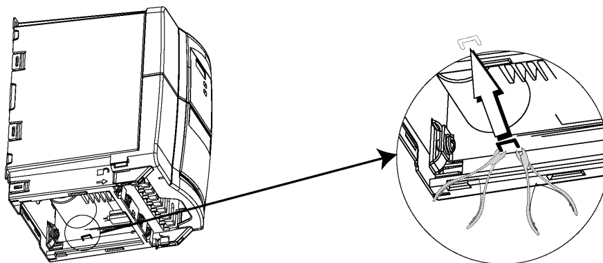
Obr. 4 Propojka Y kondenzátoru u měničů velikosti C
