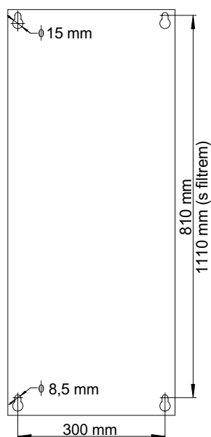
Obr. 3 Náčrtek měničů MICROMASTER 430 a vrtací předpis upevnění měničů
