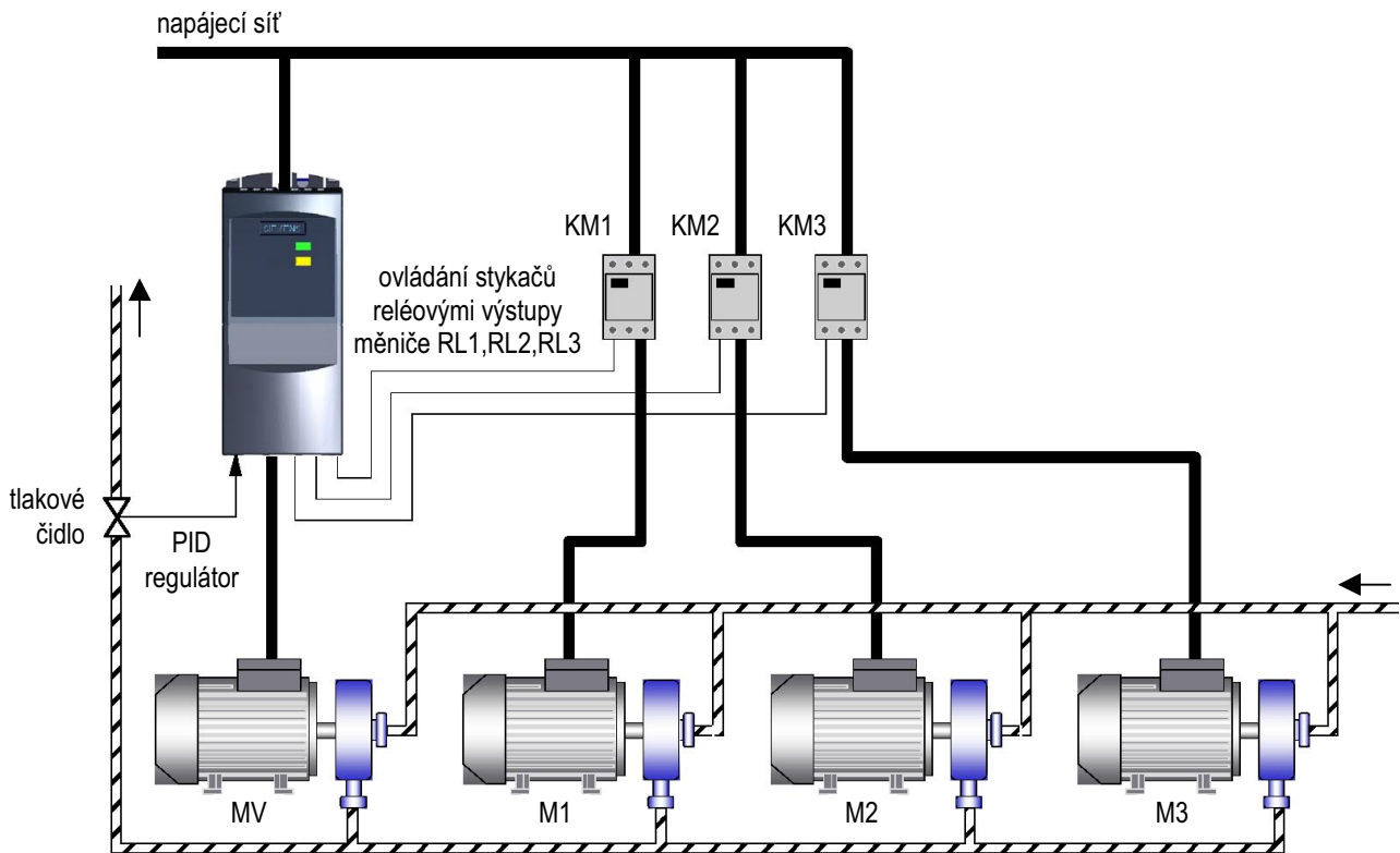
Obr. 28 Principiální schéma řízení kaskády čerpadel
