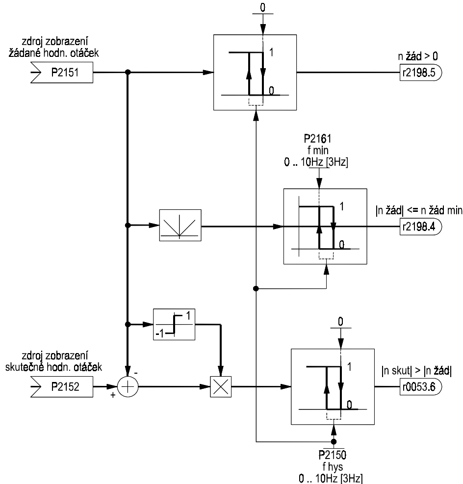
Obr. 72 Porovnání žádané hodnoty otáček
