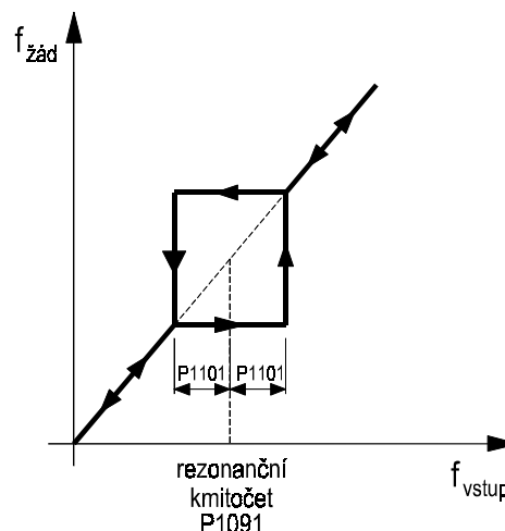
Obr. 43 Potlačení rezonančního pásma
