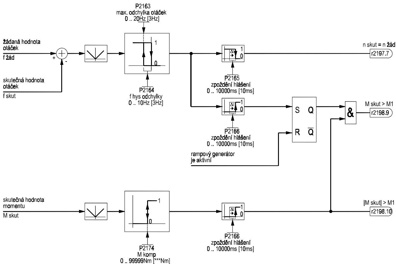
Obr. 75 Porovnání odchylky otáček
