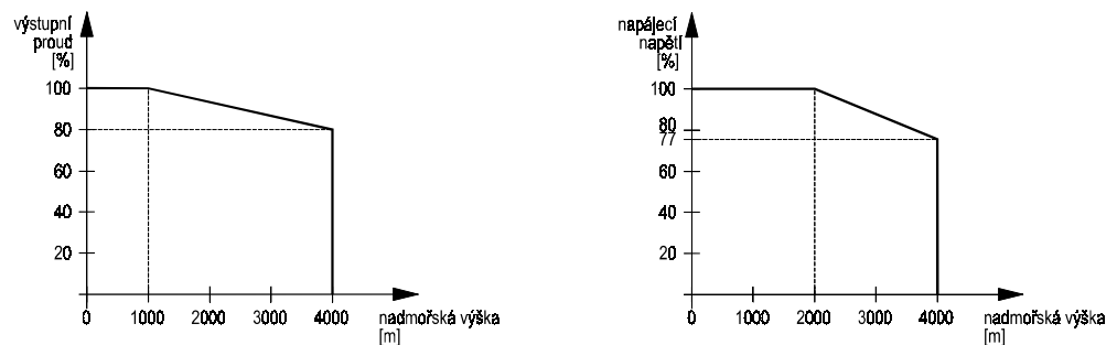
Obr. 2 Graf redukce výstupního proudu a napájecího napětí dle nadmořské výšky
