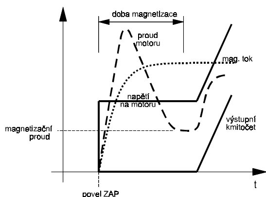
Obr. 61 Skokový nárůst magnetizačního napětí
