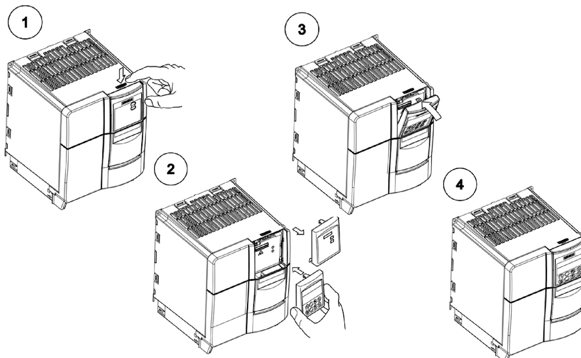
Obr. 23 Postup při výměně ovládacího panelu
