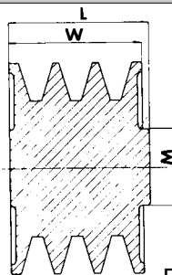
Provedení D
