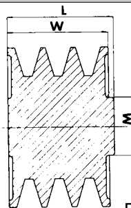
Provedení D
