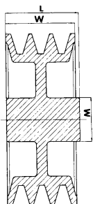
Provedení D
