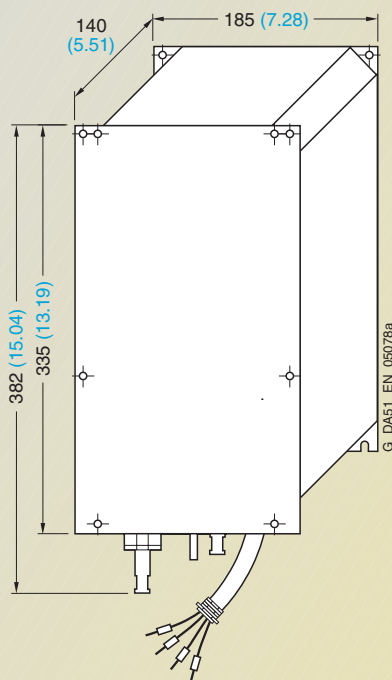
LC filtr k měničům konstrukční velikosti C 6SE6400-3TD03-2CD0
