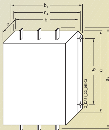
Odrušovací filtr k měničům konstrukční velikosti A
