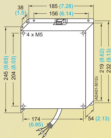
Odrušovací filtr k měničům konstrukční velikosti C
