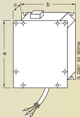
Sít'ová komutační tlumivka k měničům konstrukční velikosti B a C
