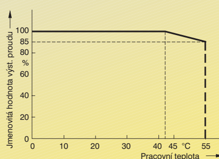
Měnič 110 až 250 kW
