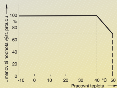
Měnič 7,5 až 90 kW
