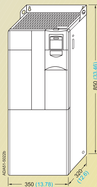
Měníč konstrukční velikosti F bez filtru
