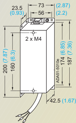
Odrušovací filtr k měničům konstrukční velikosti A
