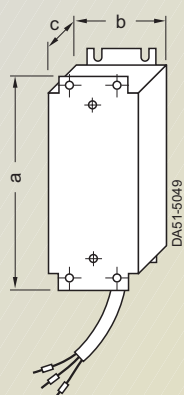
Motorová tlumivka k měničům konstrukční velikosti A 6SE6400-3TC00-4AD2 6SE6400-3TC00-4AD3
