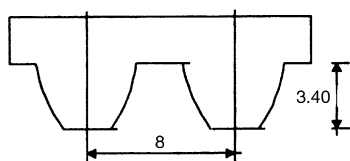
Profil Poly Chain 8MGT
