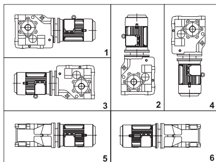
tabulka 2.3. Provedení a montážní polohy
